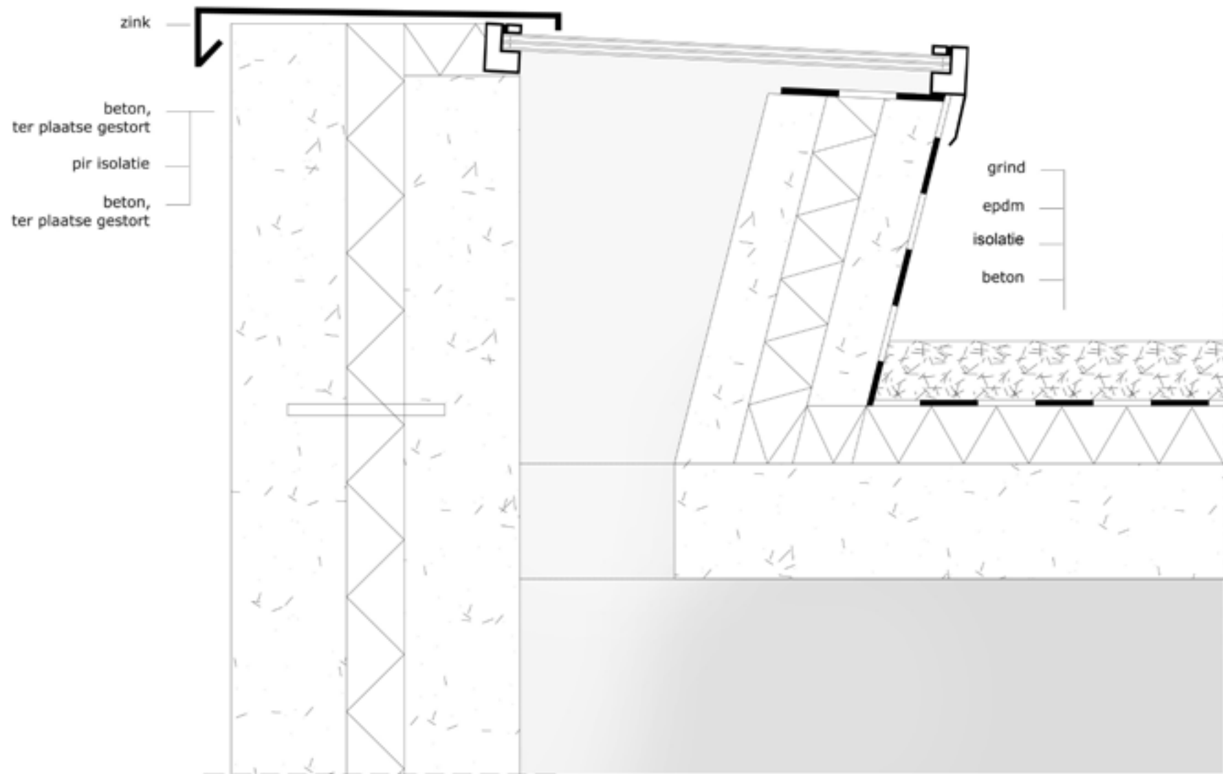
Detail bovenlicht in de rondgang naar de ceremonieruimte, 1:5
